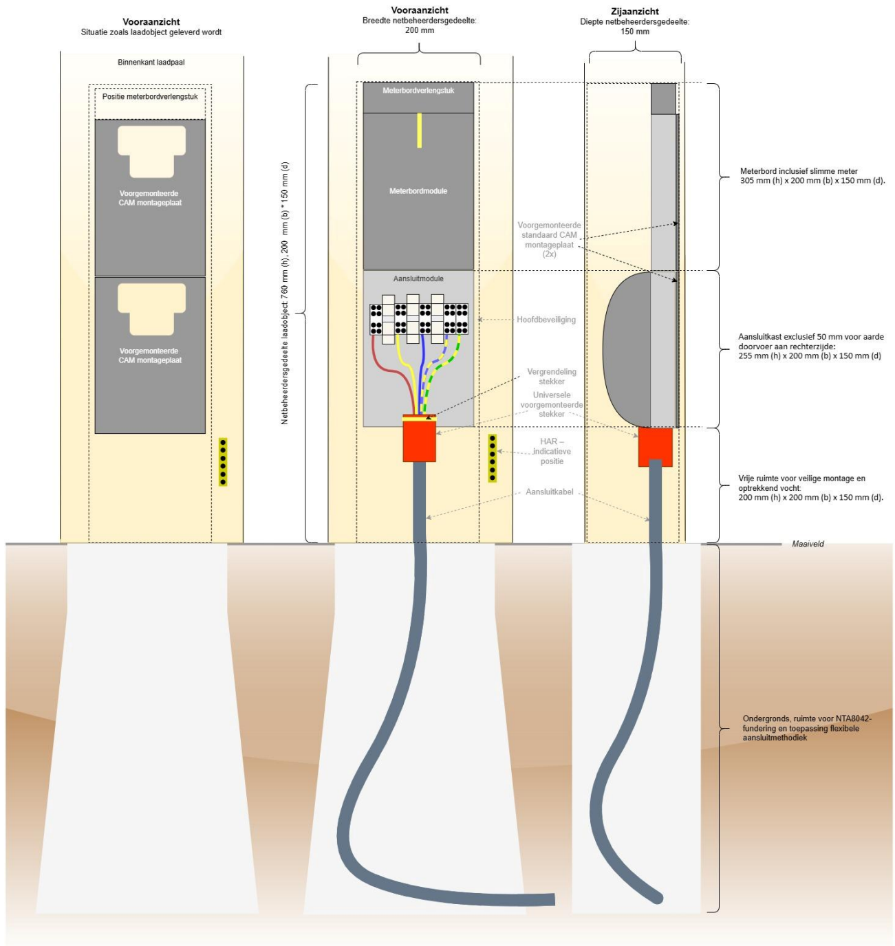
Figuur 1: inrichting en afmetingen netbeheersersgedeelte en invoer van aansluitkabel met een slimme fundering.
