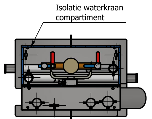
C-C ( 1 : 15 )
