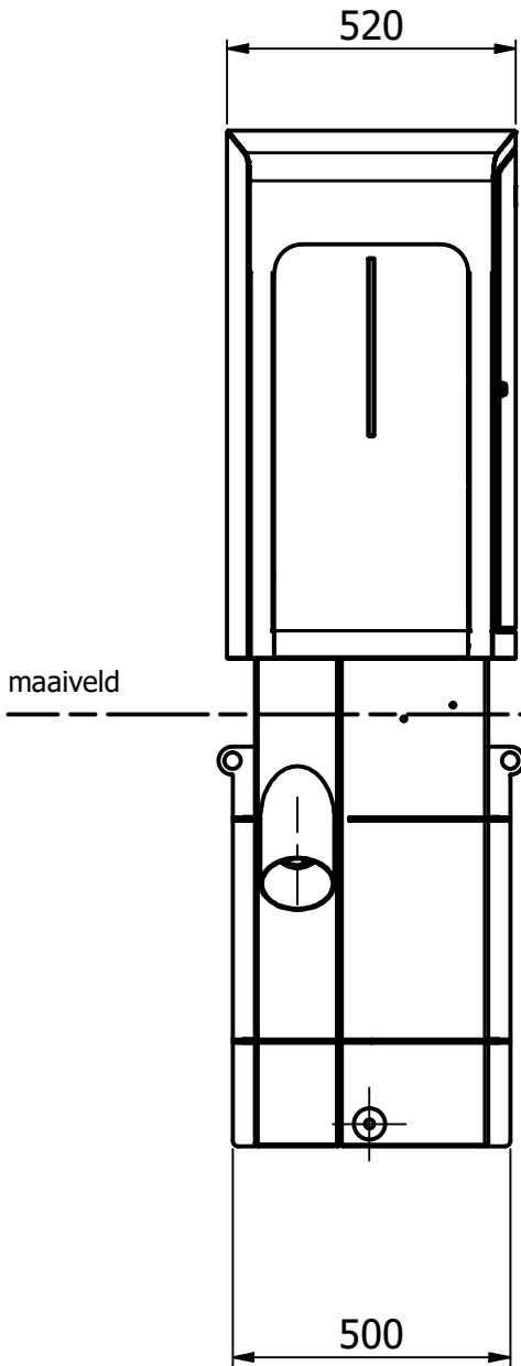
Linkerzijaaanzicht
