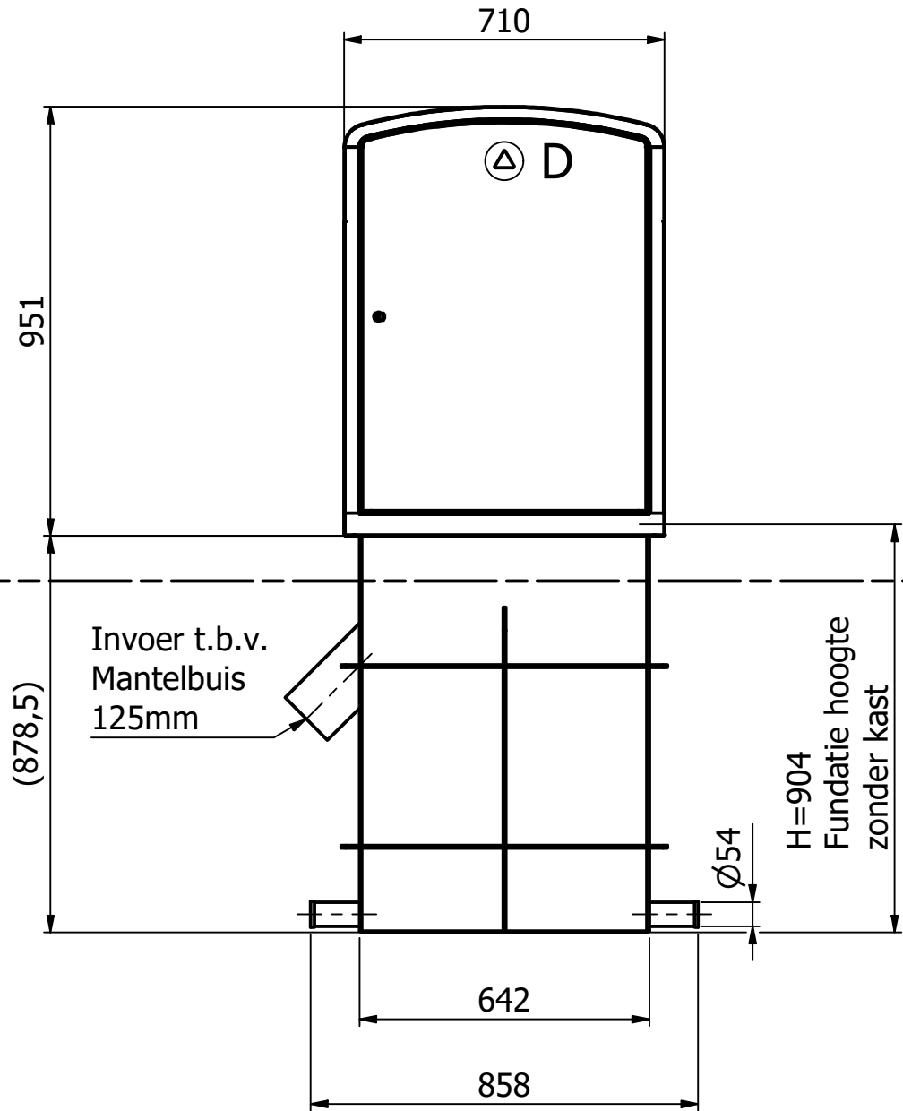
Vooraanzicht
