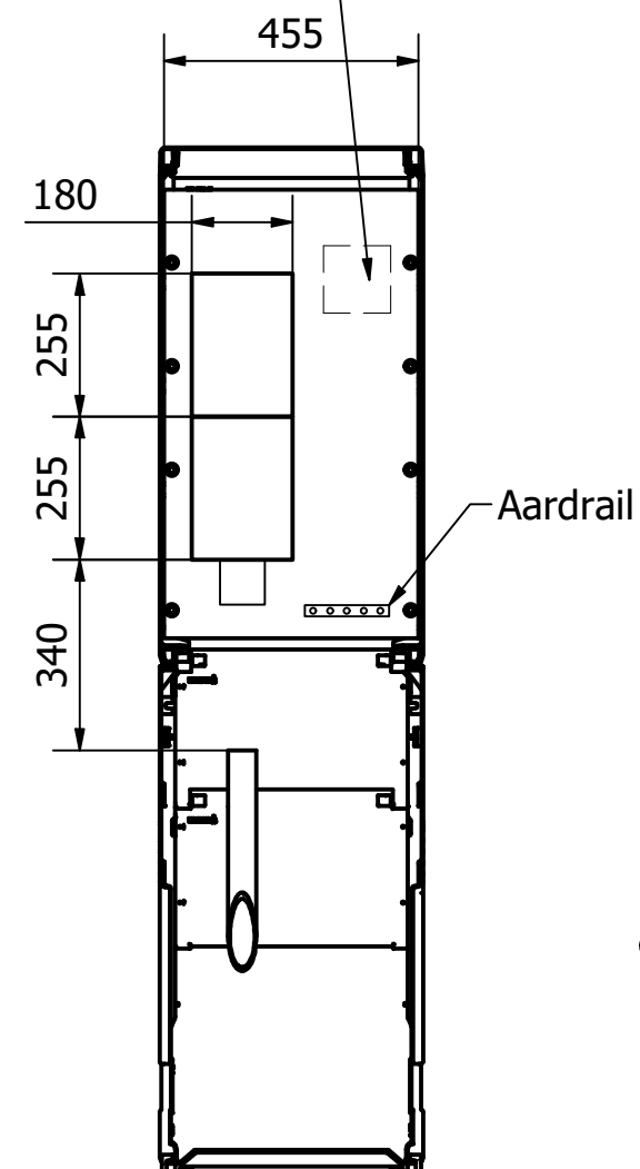
B-B ( 1:15 )
