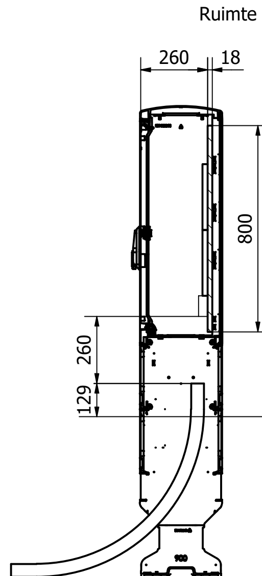
A-A ( 1:15 )
