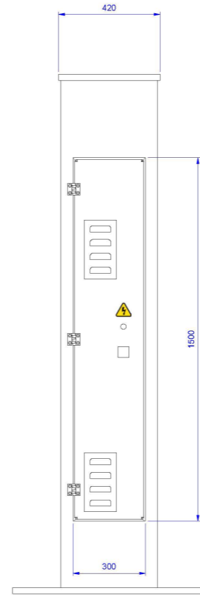
A-A (1:3)
