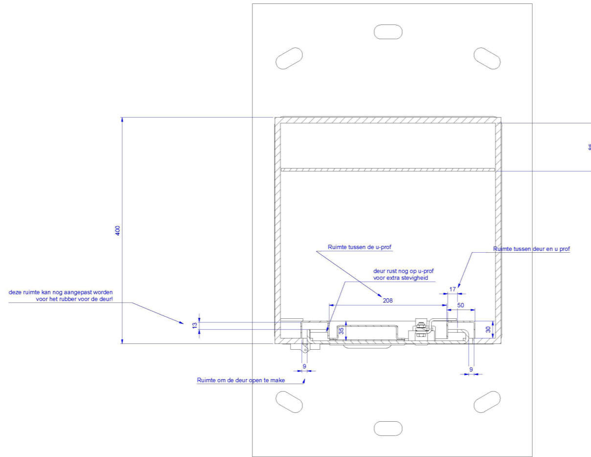
A-A (1:3)
