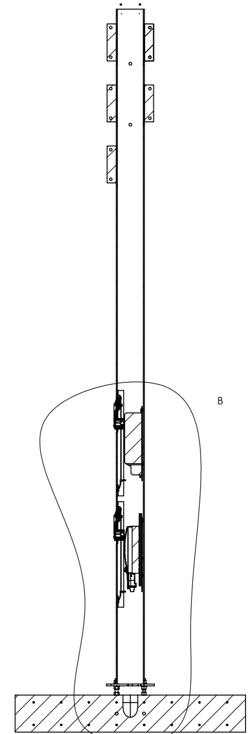
SECTION A-A
