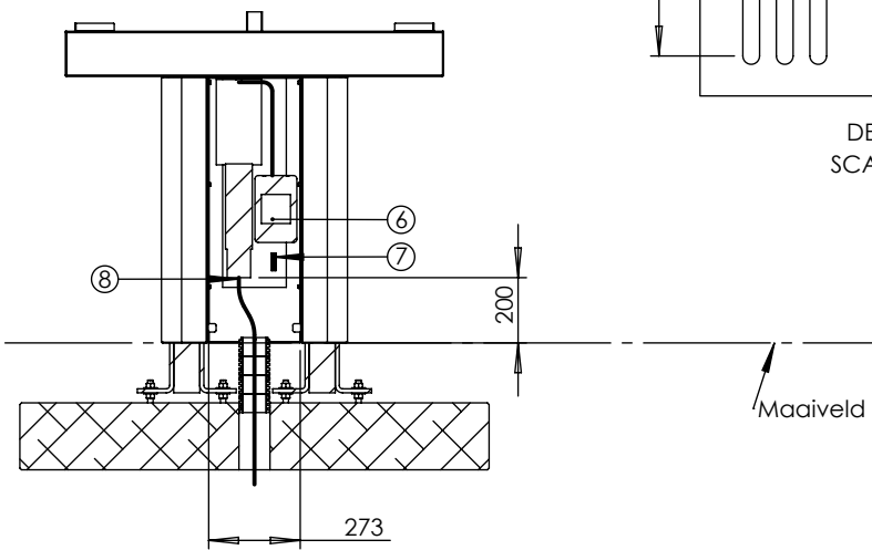
SECTION I-I SCALE 1 : 25
