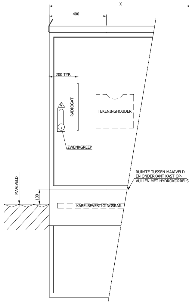
VOORAANZICHT
