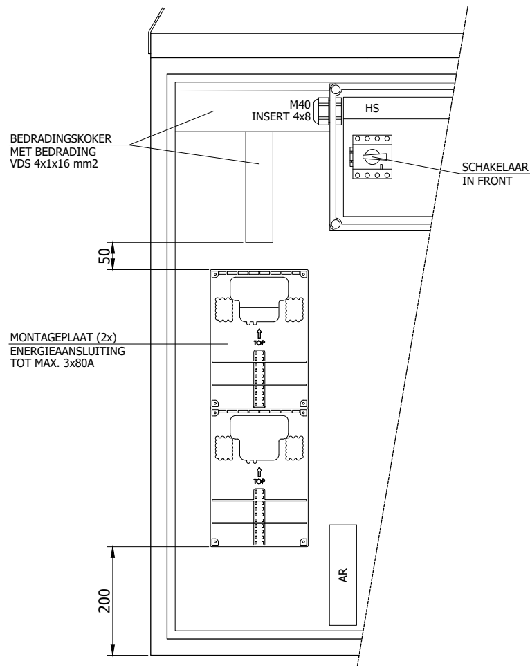
VOORAANZICHT (ZONDER DEUR EN SOKKEL)
