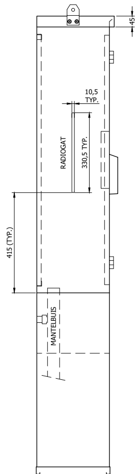
ZIJAANZICHT LINKS
