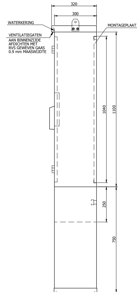
ZIJAAZICHT RECHTS
