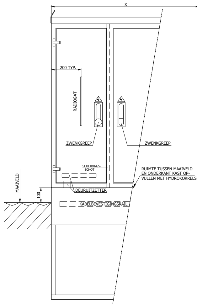
VOORAANZICHT
