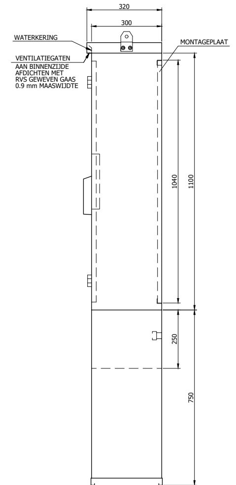
ZIJAAZICHT RECHTS
