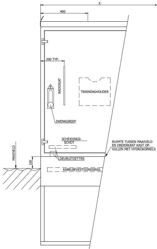
VOORAANZICHT
