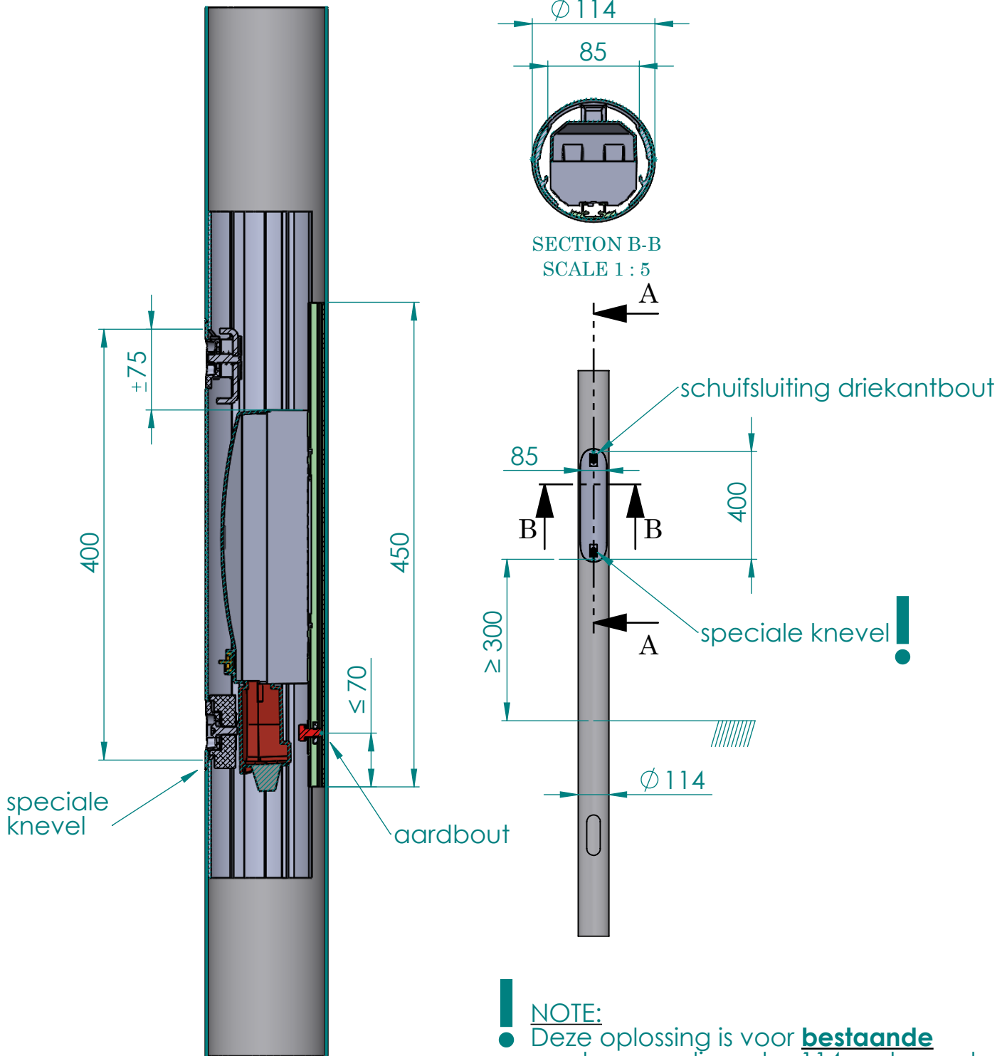
SECTION A-A SCALE 1 : 5
