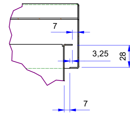
E (1:3) Ventilatie
